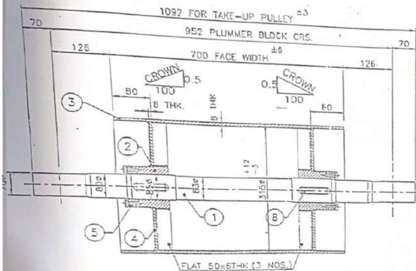
ELEVATION
